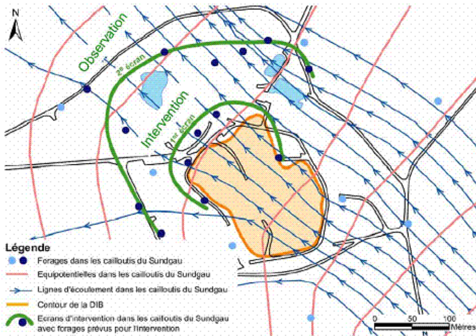
Emplacement des forages de surveillance de l'aquifère (cailloutis du Sundgau)
