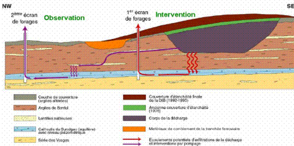
Coupe géologique avec les barrières d'intervention et d'observation
