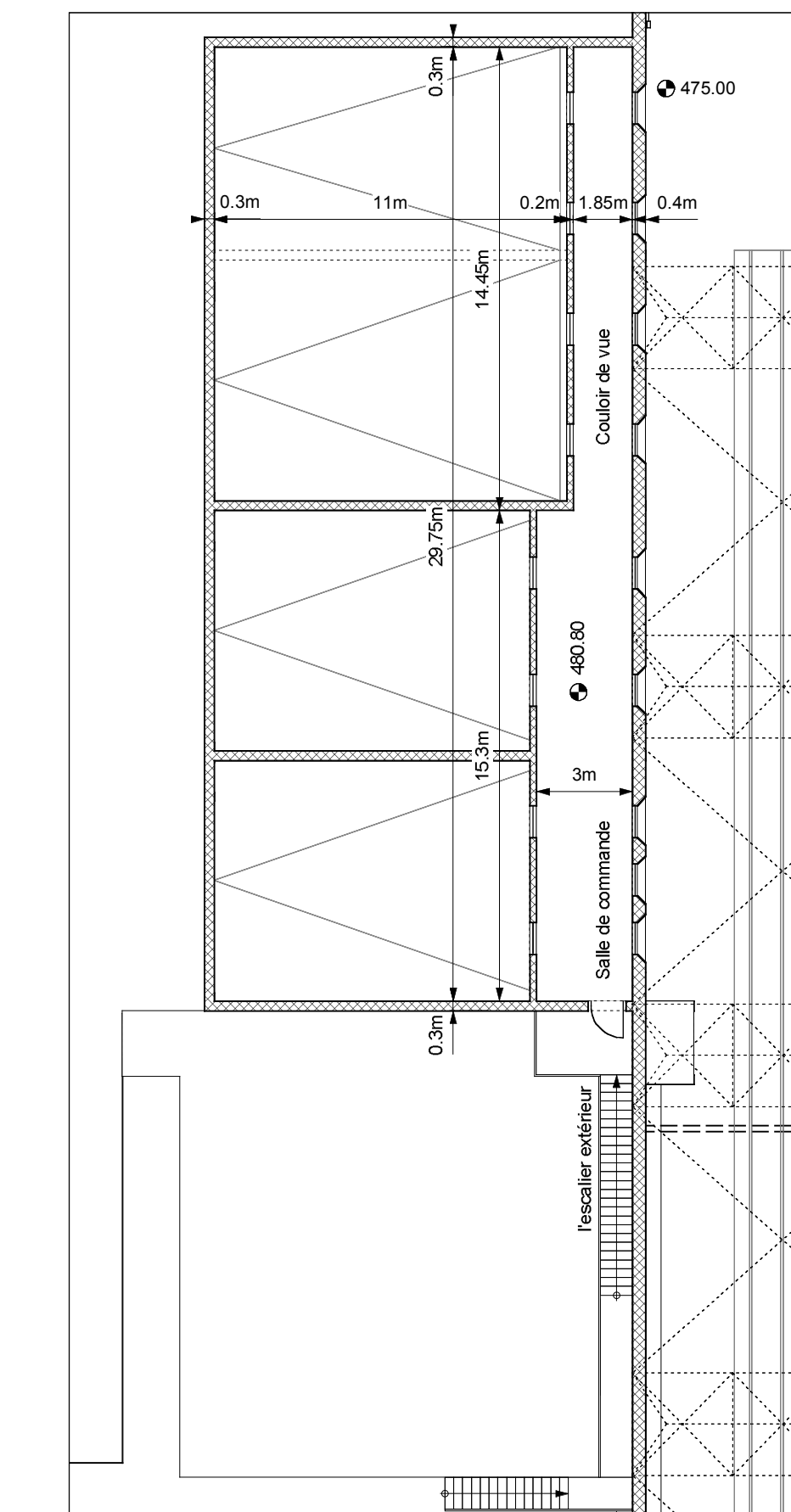
Salle de commande, vue en plan 1:200, niveau + 481.00
