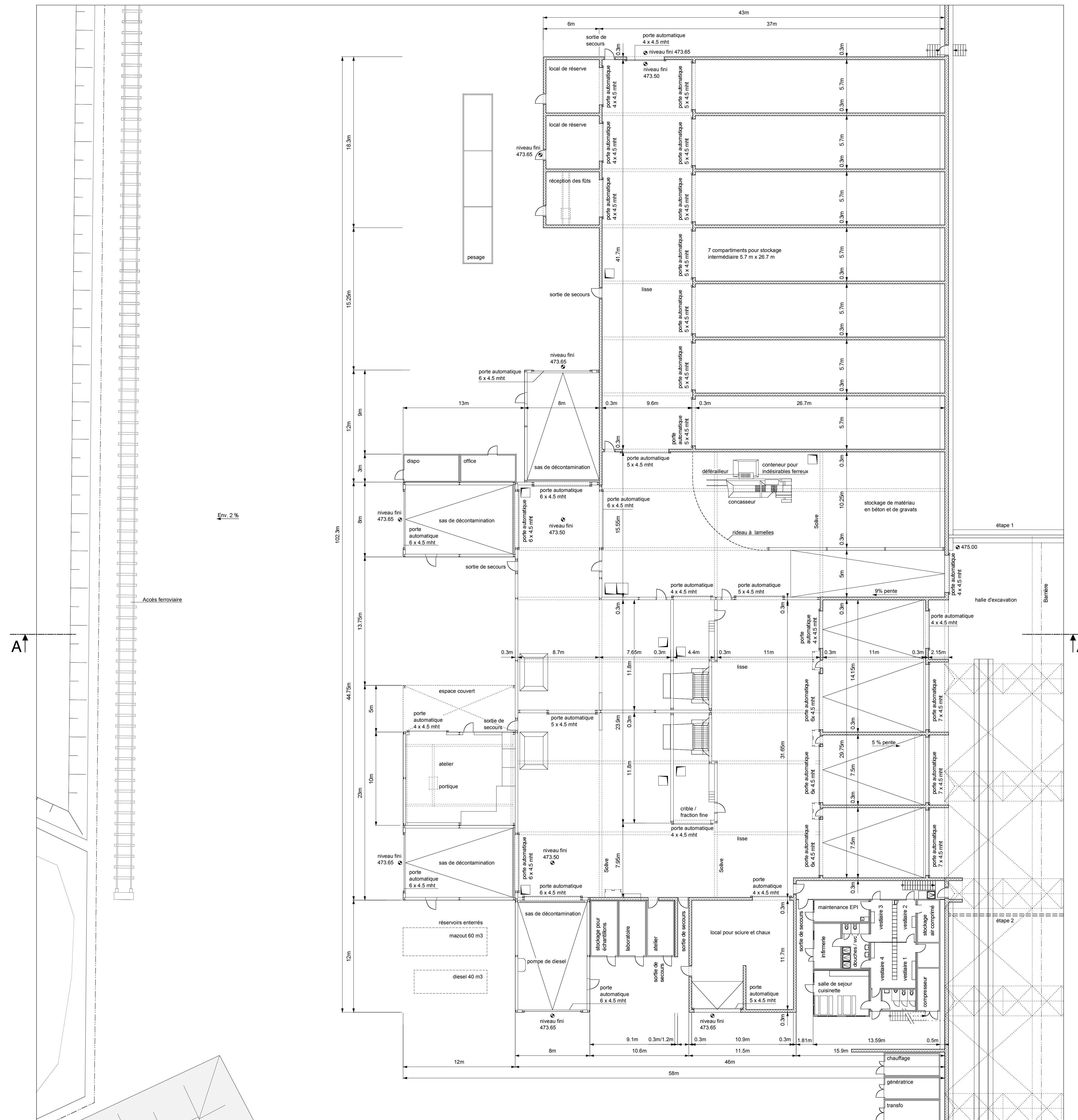
Vue en plan 1:200, niveau + 476.50
