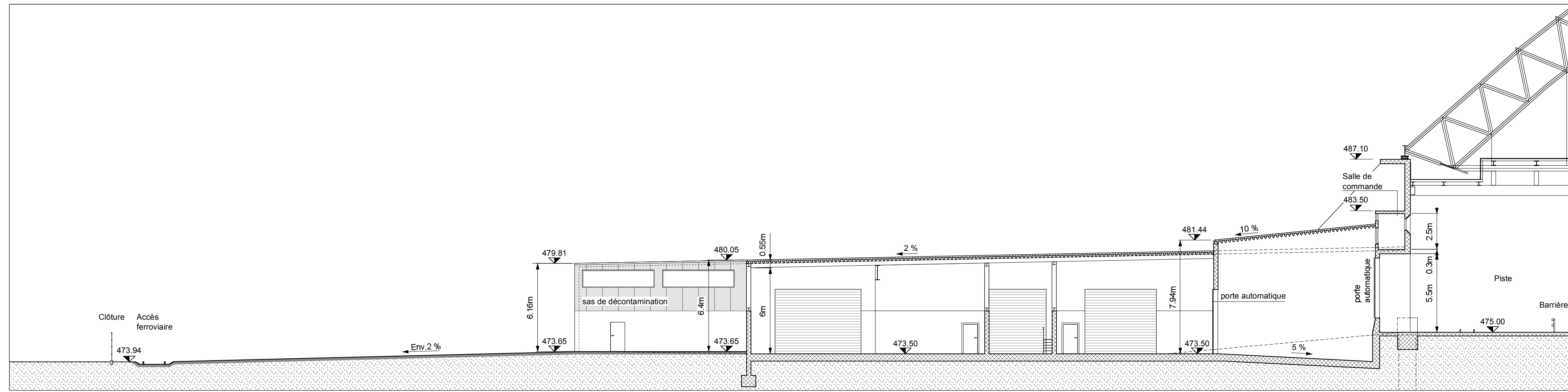
Coupe A-A 1:200
