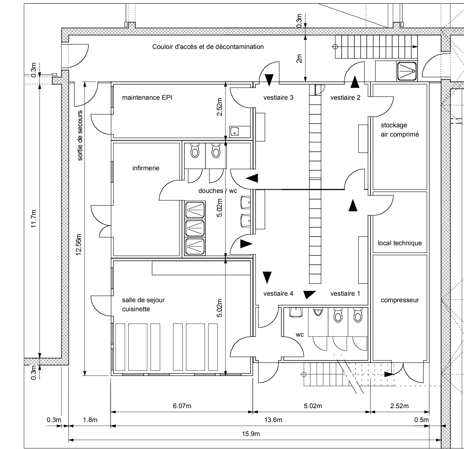
Secteur noir/blanc, vue en plan 1:100, niveau + 475.50
