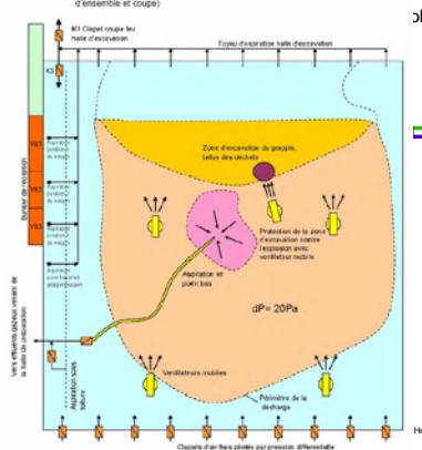
Fig. 2.1 Redevance de ventilation isolante dans la halle d'excavation (plan schématisé d'ensemble et coupe)
