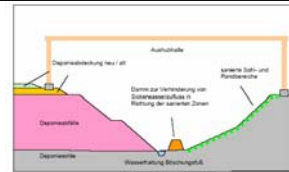
Abbildung 28 Schema Dachneubauechtung / Wasserhaltung
