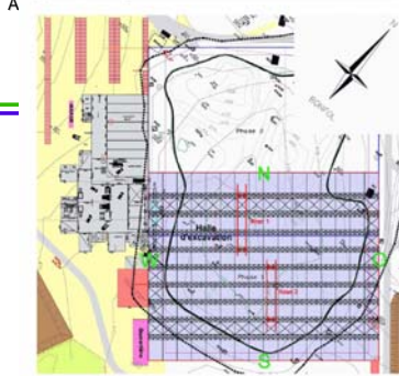
Fig. 3.2 Plan de situation avec la halle d'excavation (étape 1, filas) et la halle de préparation (gris) de la CIB. Les lignes de niveau du couvercle de la décharge sont représentées en noir, celles de la base de la décharge en vert foncé. Les lettres vertes O, E, N, S désignent les quatre façades de la halle d'excavation.
