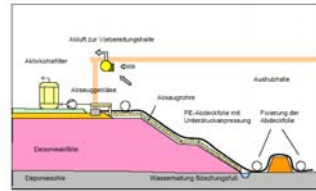
Abbildung 30 Unterdruckabdichtung mit Abluftabgang
